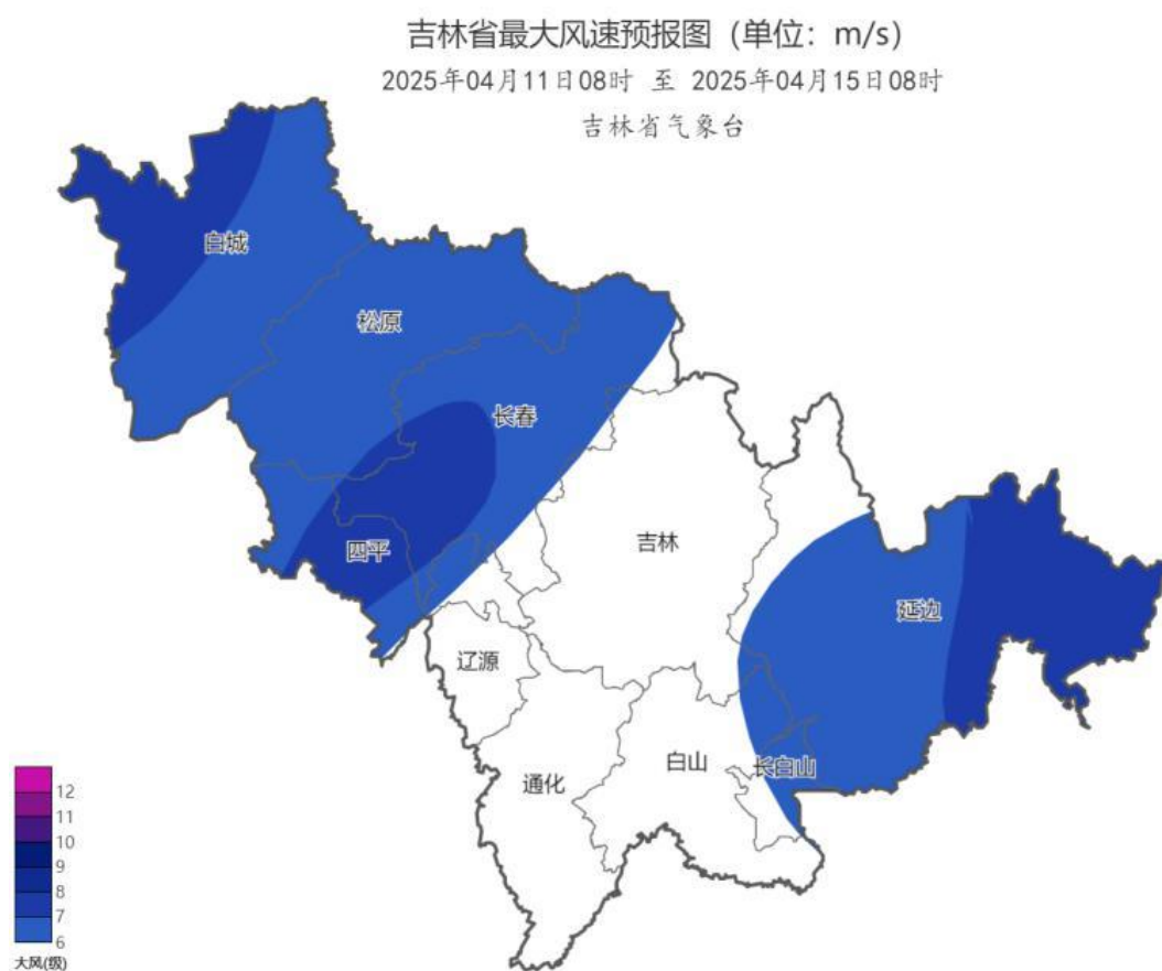
图1 吉林省最大风速预报图
