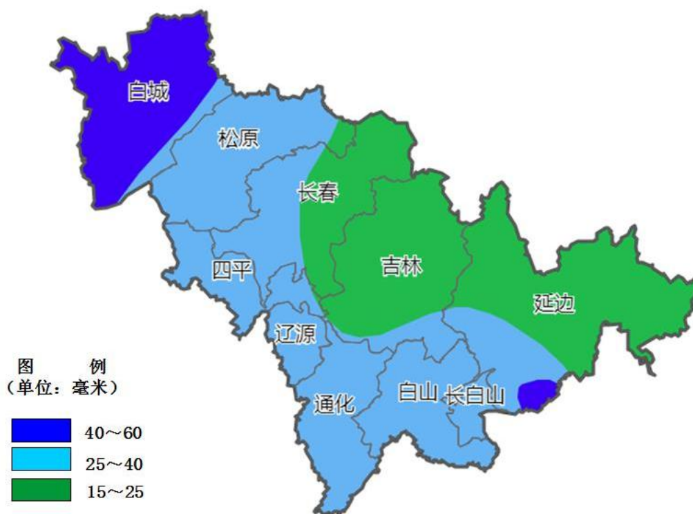
图 2 4 月 11 日午后-15 日降水量预报图
